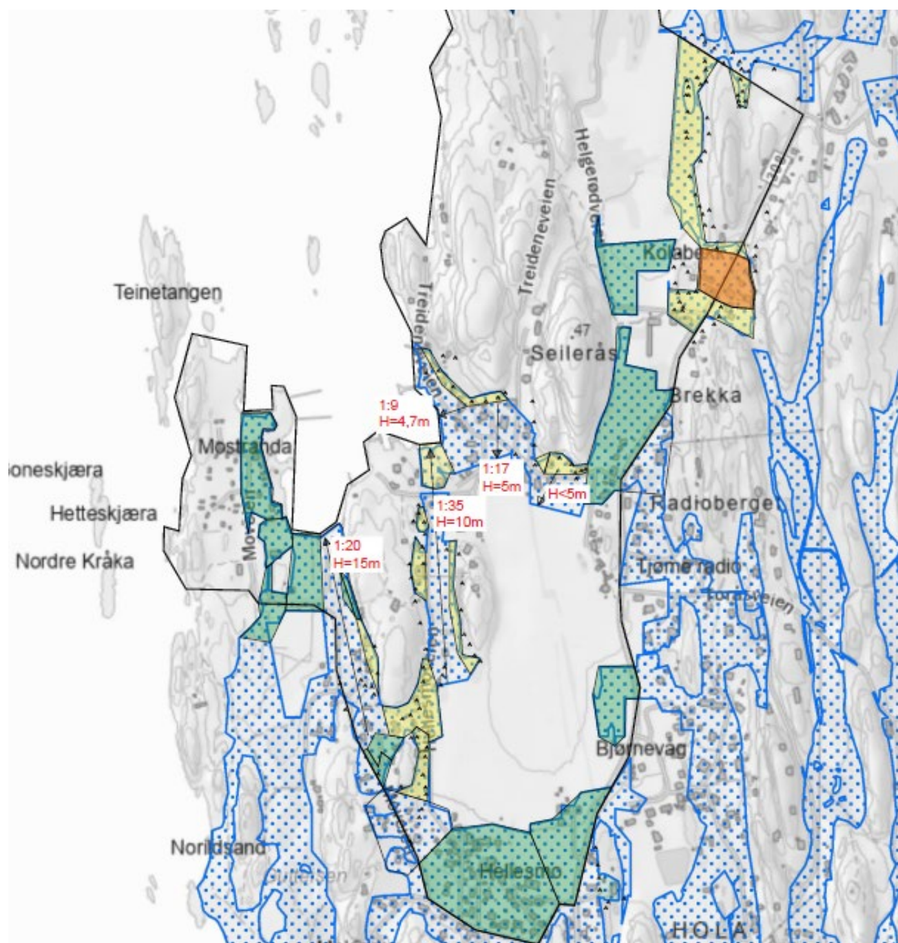
Figur 2: Utklipp fra tegning 116744-38 Mulig faresone er markert med oransje. Gule områder viser områder hvor befarings utført, og grønne områder er vurdert som trygge med bakgrunn i høydeforskjell/terrengkriteriet.
