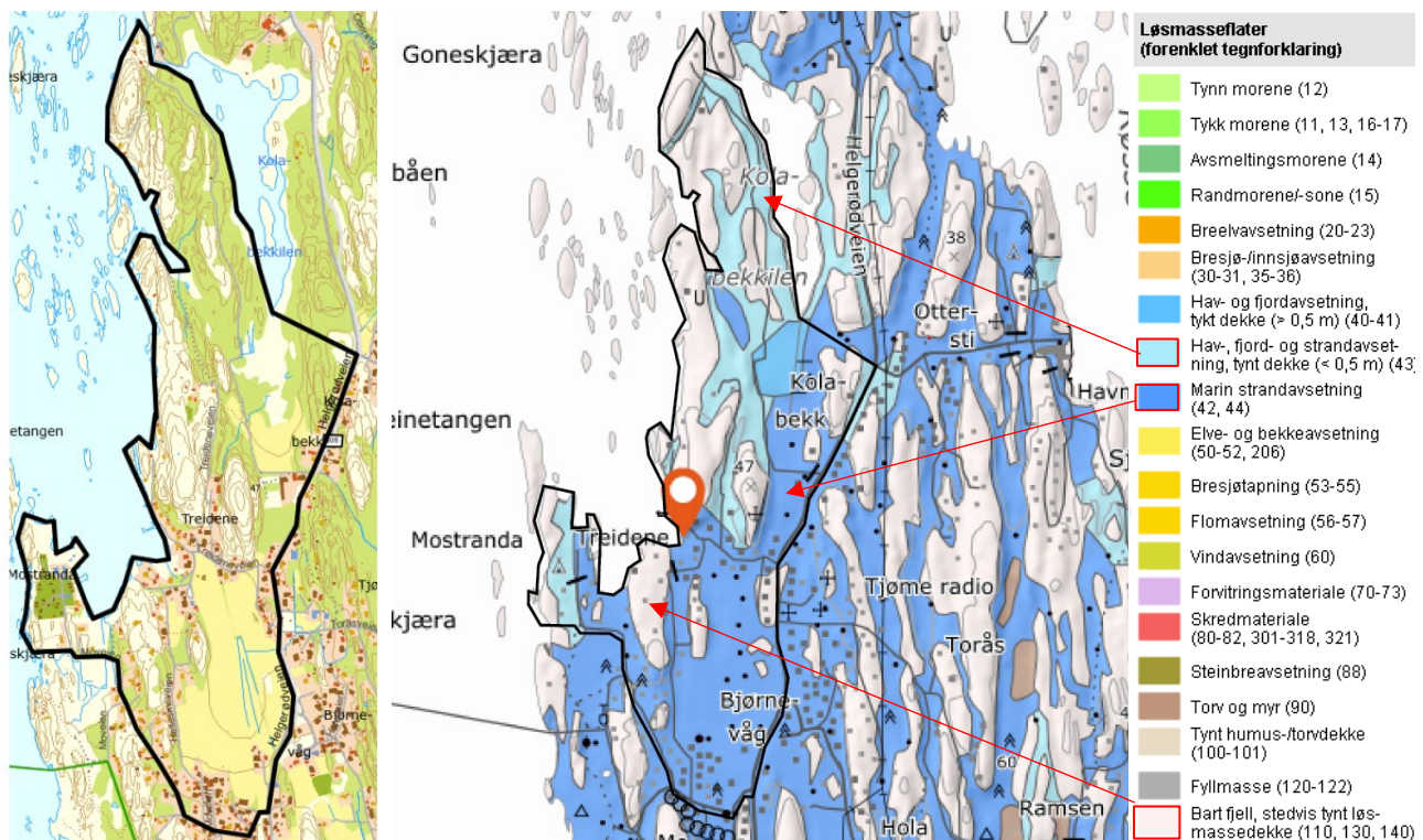
Figur 1: Delområde 34 på mottatt kart fra Færder kommune (venstre) og Kvartærgeologisk kart fra www.ngu.no (høyre).
