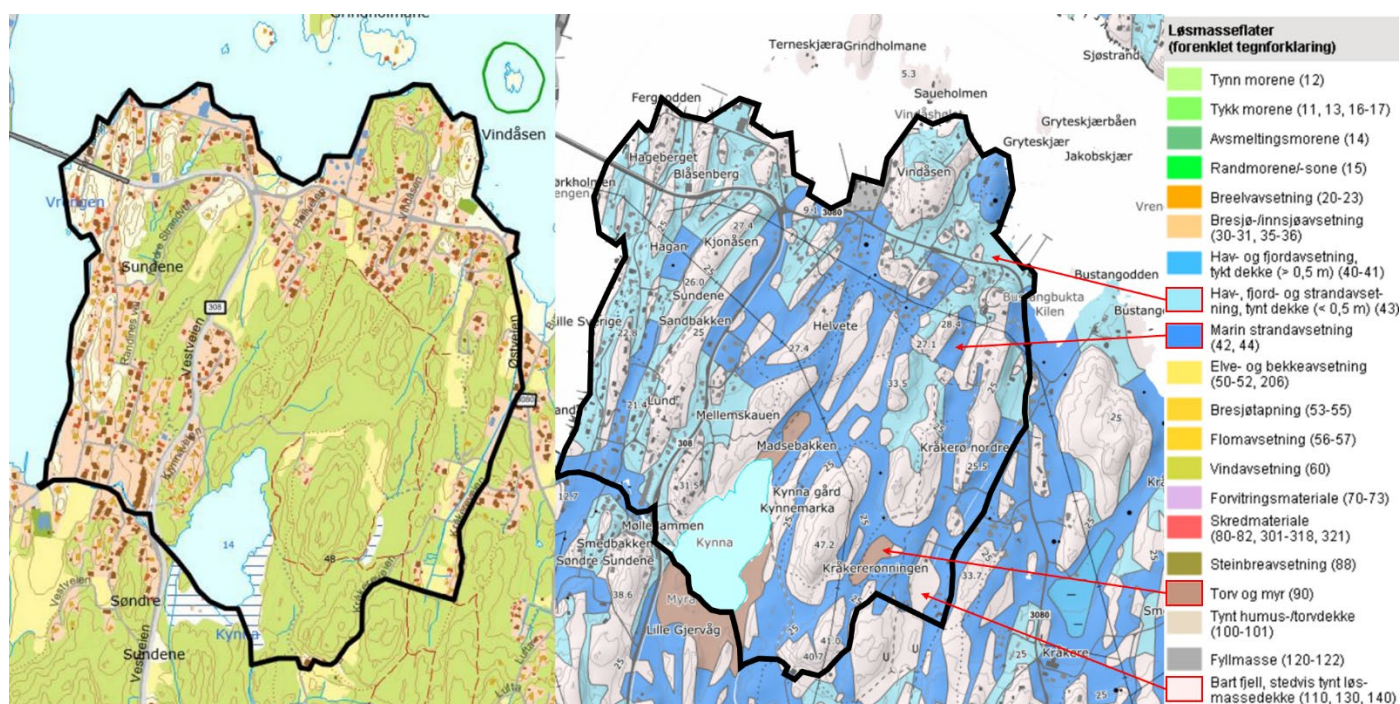
Figur 1: Delområde 37, på mottatt kart fra Færder kommune (venstre) og Kvartærgeologisk kart fra www.ngu.no (høyre).
