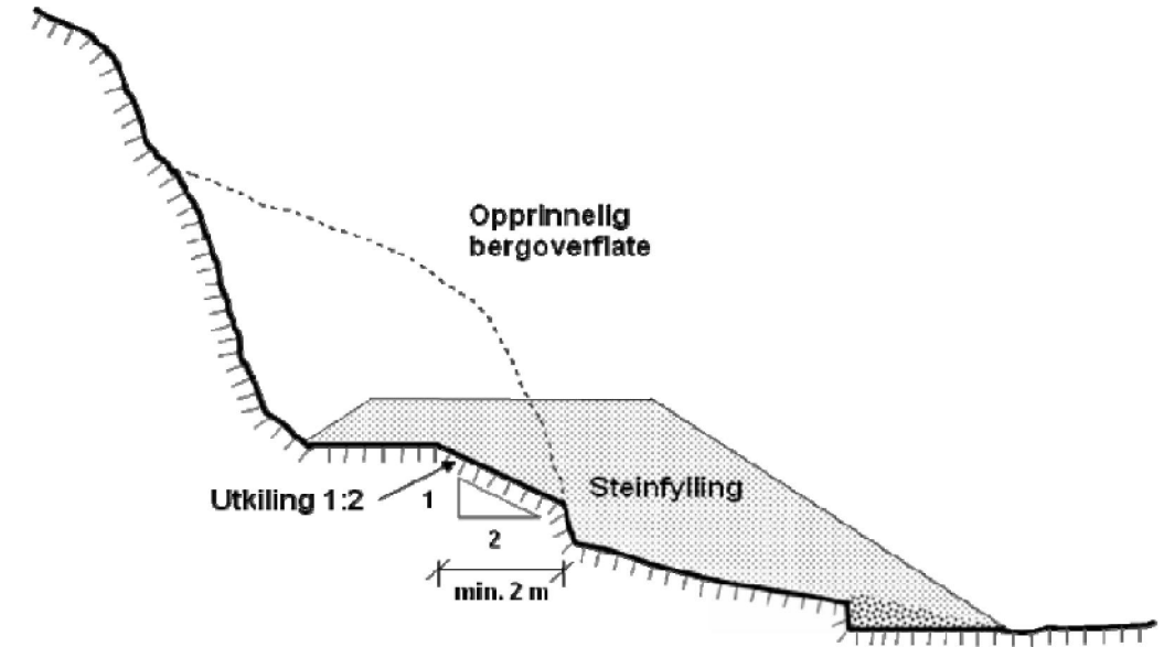
UTKILING I OVERGANG MELLOM STEINFYLLING OG STEINSKJÆRING
