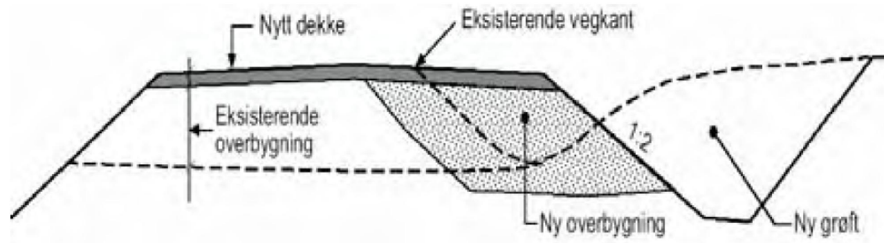
UTKILING VED UTVIDELSE AV VEI
