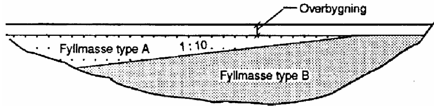
UTKILING AV MASSER I FYLLING (LENGDEPROFIL)
