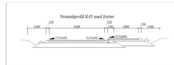
Figur 1- Planlagt Tverrprofil
