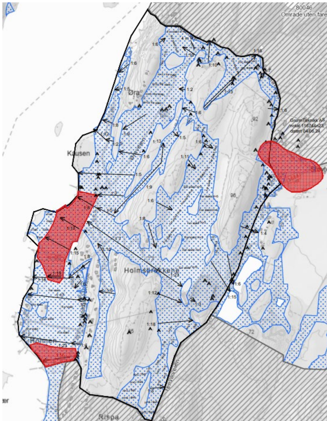
Figur 2: Utklipp fra tegning 116744-50. Gjenværende aktsomhetsområder er markert med rød skravur.
