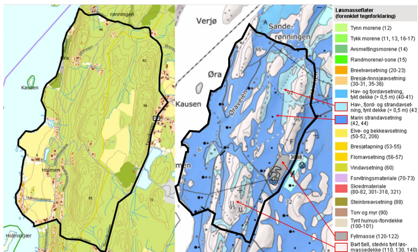
Figur 1: Delområde 43 på mottatt kart fra Færder kommune (venstre) og Kvartærgeologisk kart fra www.ngu.no (høyre).
