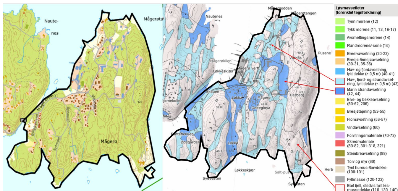
Figur 1: Delområde 46 på mottatt kart fra Færder kommune (venstre) og Kvartærgeologisk kart fra www.ngu.no (høyre).
